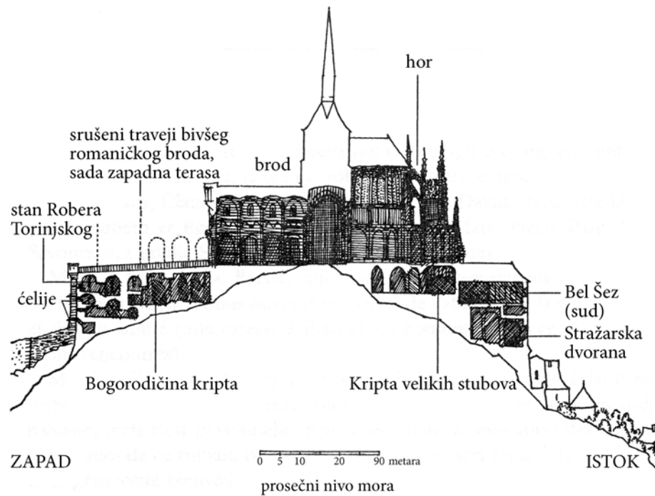
Uzdužni presek Mon Sen Mišela (od zapada prema istoku) po E. Korojeju
